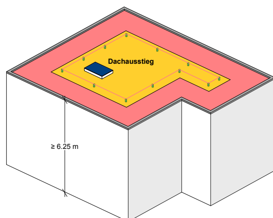
Abb. 13: Ausstattungsklasse 1: EAP am Dachrand entlang der Geometrie des Gebäudes angepasst. Kontrolle wird mit einem temporärem Seilsystem ausgeführt
