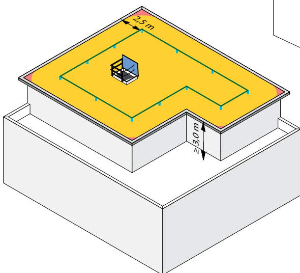
Abb. 15: Ausstattungskategorie 2: Permanentes Seilsystem bei geringem Sturzraum einsetzen, z. B. bei Attikaterassen oder bei Bauten mit Höhen unter 6,25 m
