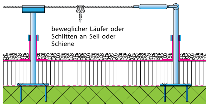
Abb. 14: Ausstattungskategorie 2: permanentes horizontales überfahrbares Seilsystem mit Spannvorrichtung, direkt in Stahlbeton verankert
