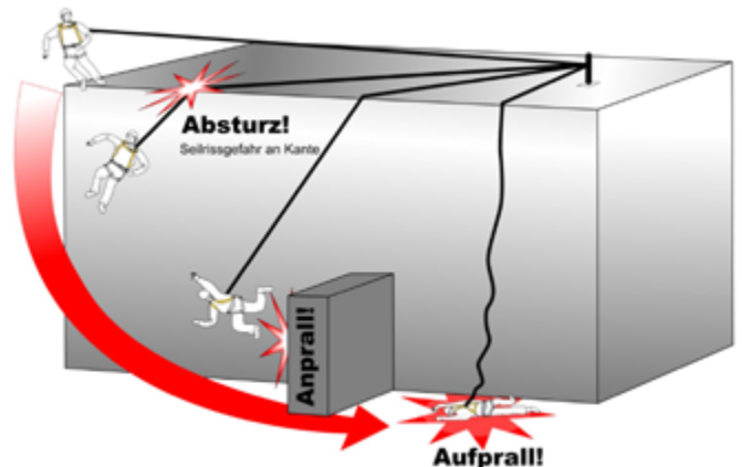
Abb. 34: Gefahren bei einem Pendelsturz
