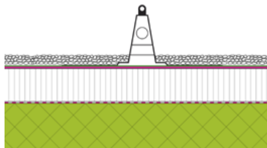
Abb. 6: Ausstattungskategorie 1; EAP auf einem wärmedämmten Flachdach eingebaut, Variante auf der Abdichtung mit Substrat beschwert. (Herstellerangaben beachten, Wintertauglichkeit abklären)
