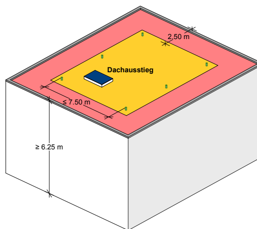
Abb. 8: Regelabstand von EAP
