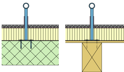
Abb. 5: Ausstattungskategorie 1: EAP auf einem wärmedämmten Flachdach eingebaut, Variante auf einer Beton- und einer Holzunterkonstruktion
